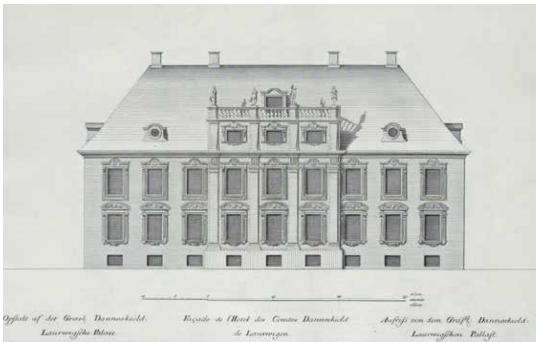
Kobberstik af Danneberg-Laurvigs Palæes facade fra Thurahs Den Danske Vitruvius. Foto: The Getty Research Institute.
