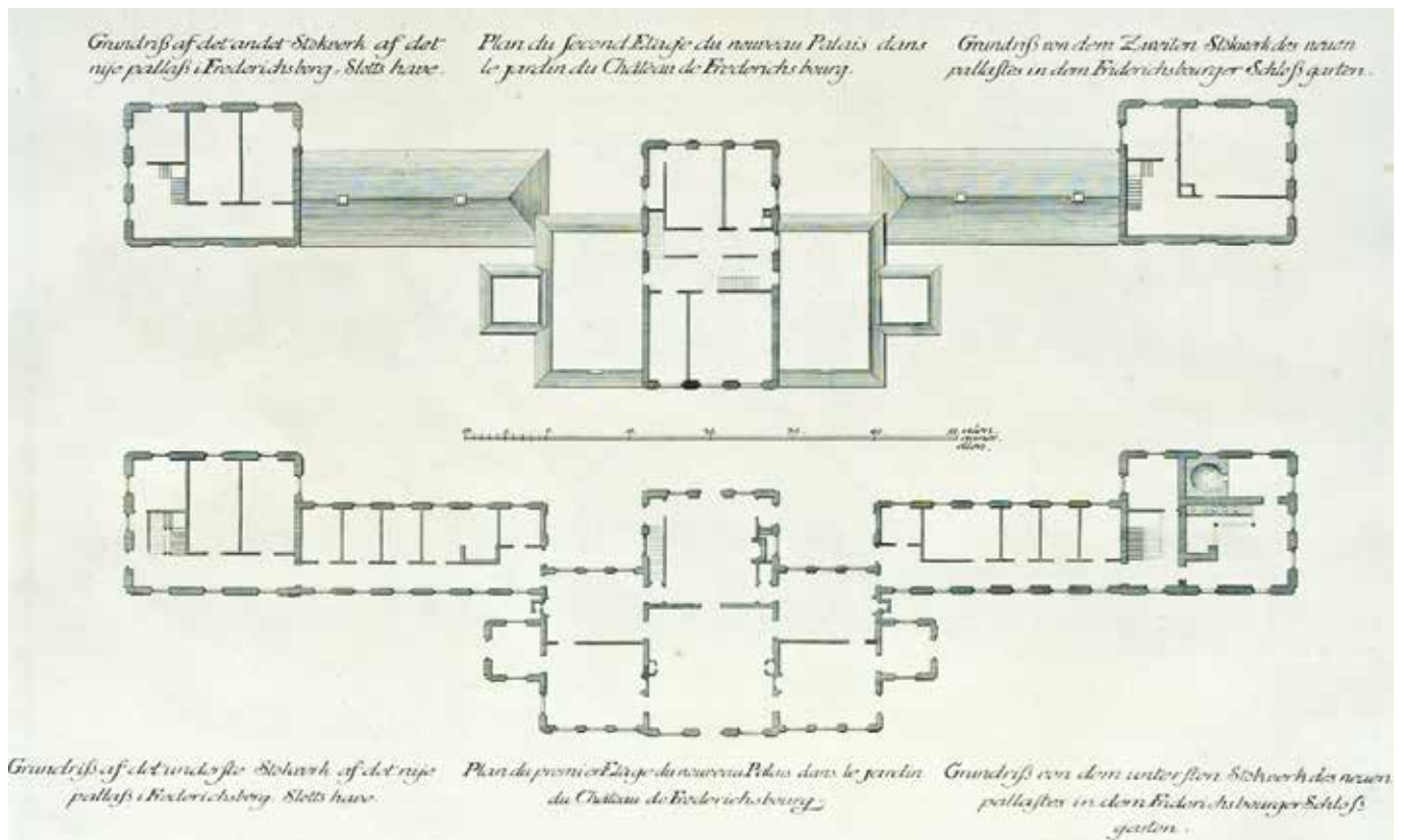
Grundplan over Det Kinesiske Hus i Thurahs Den Danske Vitruvius. Foto: The Getty Research Institute.
